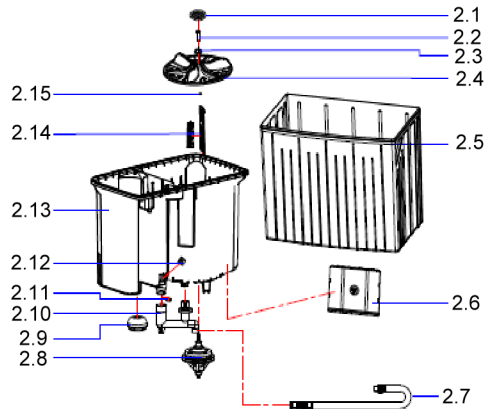
2:Cabinet Subassembly
