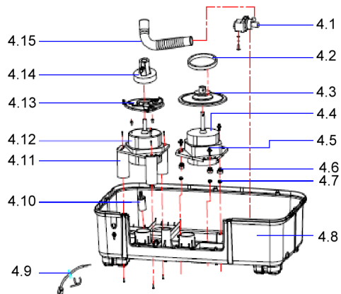
4:Base Subassembly
